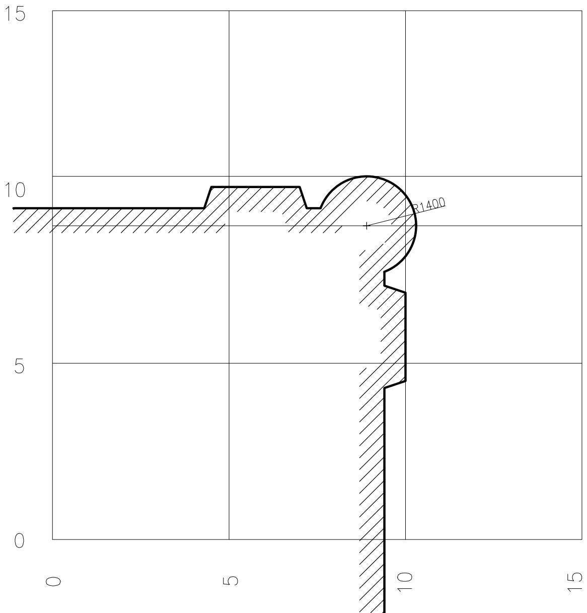
ПРОФИЛЬ 5 МАСШТАБ 1:1
