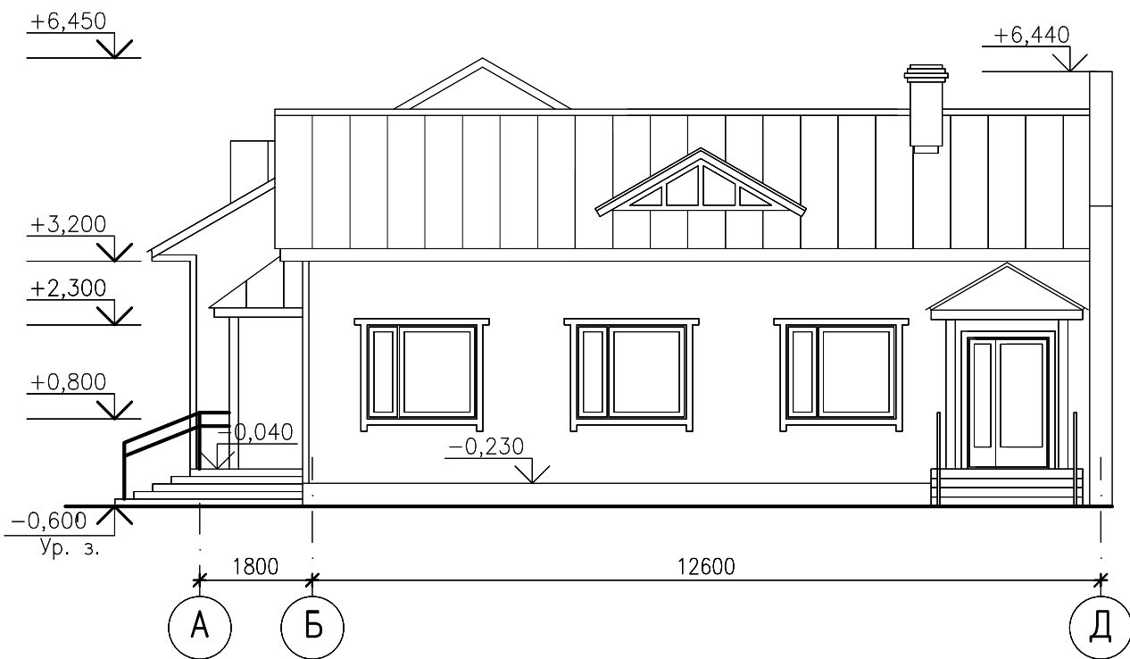
ФРАГМЕНТ ФАСАДА КАРКАСНОГО ЗДАНИЯ
