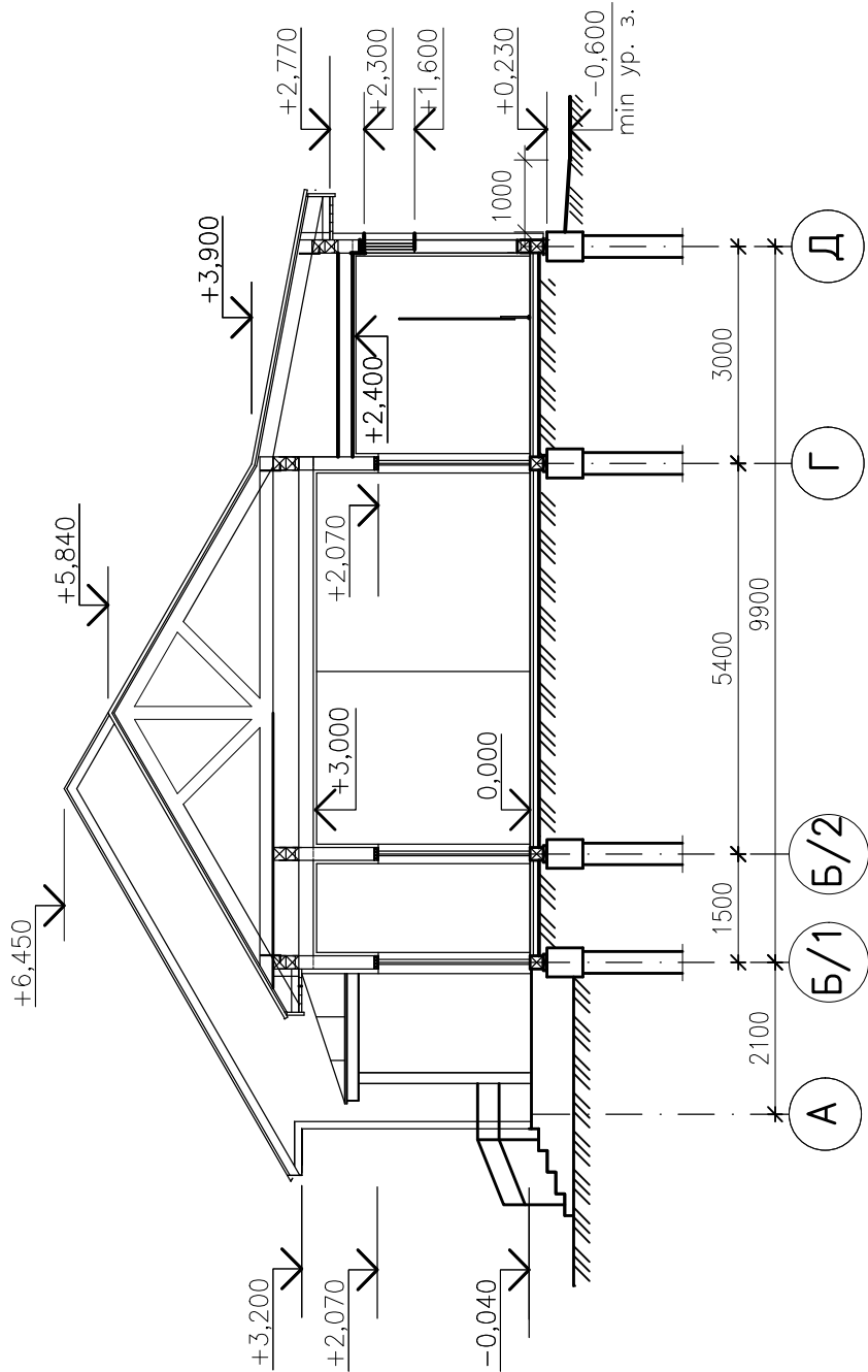
РАЗРЕЗ 3-3
