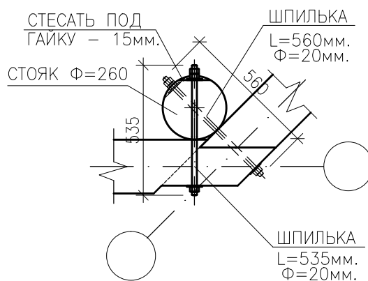
УЗЕЛ 10 (УСТАНОВКА СТОЯКА В УГЛАХ)
