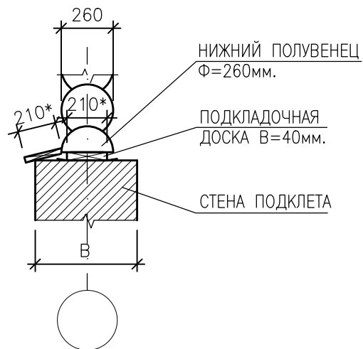
УЗЕЛ 8 (ПОПЕРЕЧНАЯ СТЕНА)
