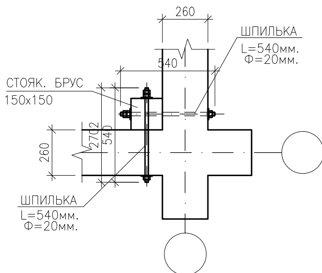
УЗЕЛ 9 (УСТАНОВКА СТОЯКА В УГЛАХ)
