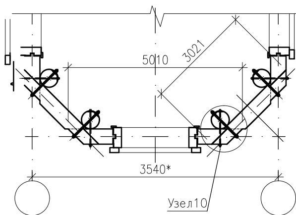
СОПРЯЖЕНИЯ ВЕНЦОВ В ЛАПУ
