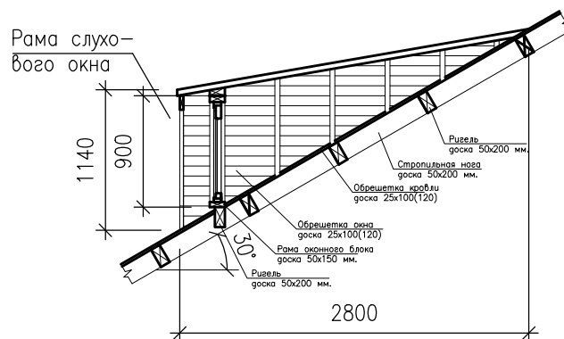
РАЗРЕЗ 1-1
