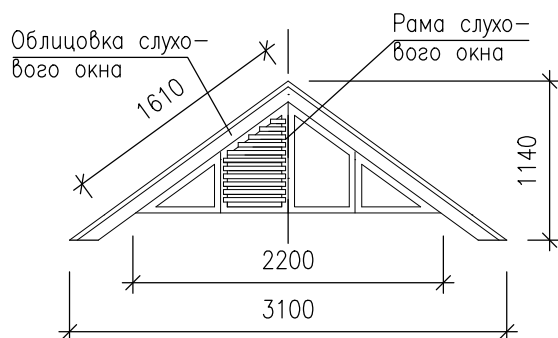
ФАСАД
