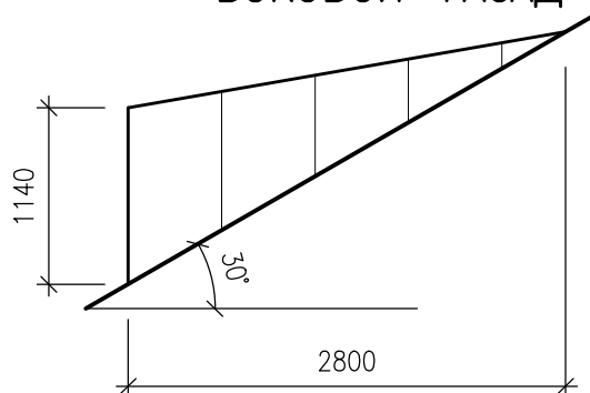
БОКОВОЙ ФАСАД
