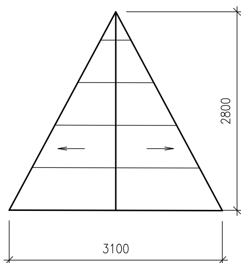
ПЛАН КРОВЛИ
