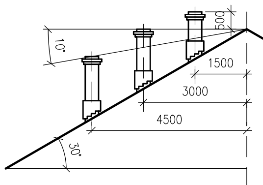
РАСПОЛОЖЕНИЕ ДЫМОВЫХ ТРУБ ОТНОСИТЕЛЬНО КОНЬКА КРЫШИ
