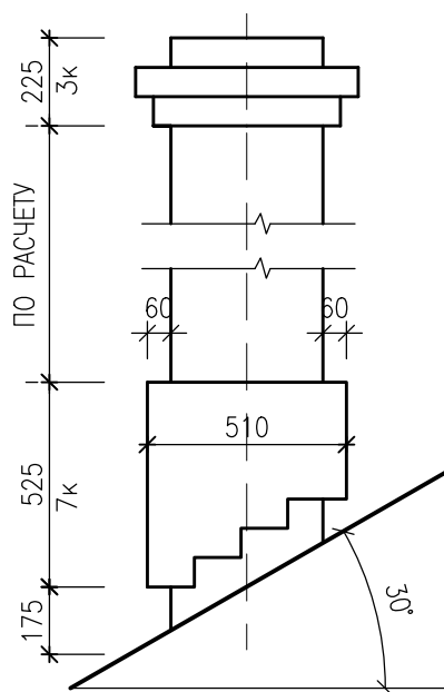
БОКОВОЙ ФАСАД
