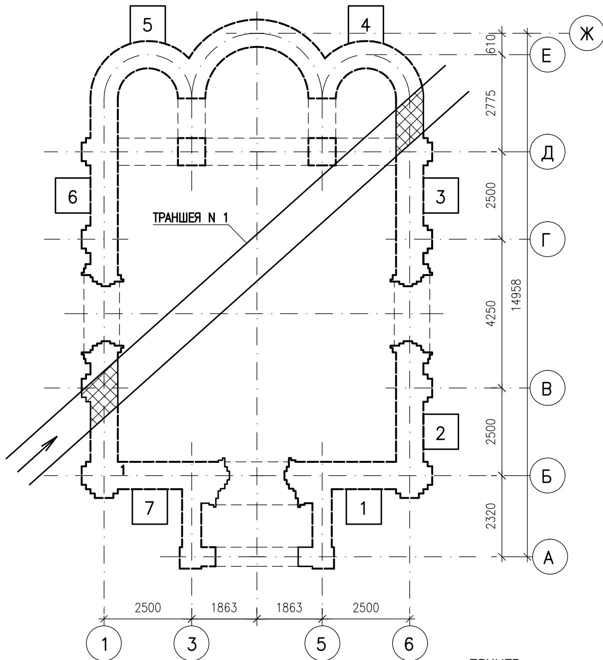
ПРИМЕР КОНСЕРВАЦИЯ ВЕРХНЕГО ОБРЕЗА СТЕН РУИН
