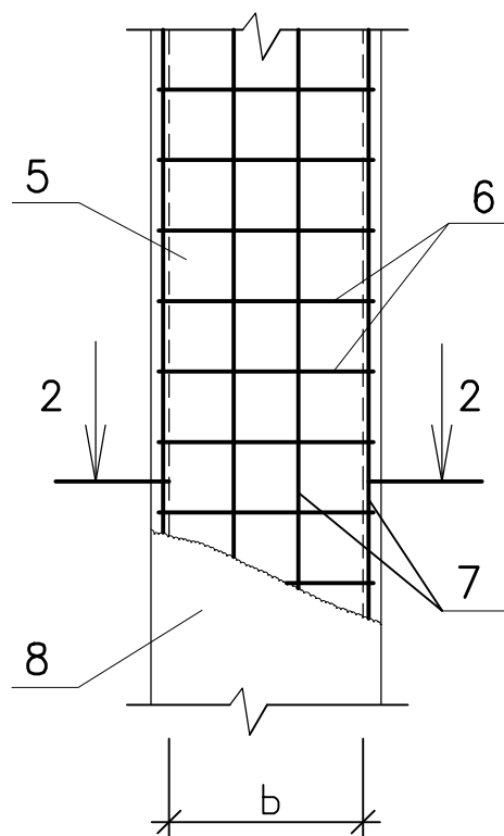
2.СХЕМА УСИЛЕНИЯ СТОЛБОВ И ПРОСТЕНКОВ ОБОЙМАМИ (Бетон)
