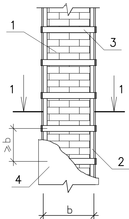
1.СХЕМА УСИЛЕНИЯ СТОЛБОВ И ПРОСТЕНКОВ ОБОЙМАМИ (Кирпич)
